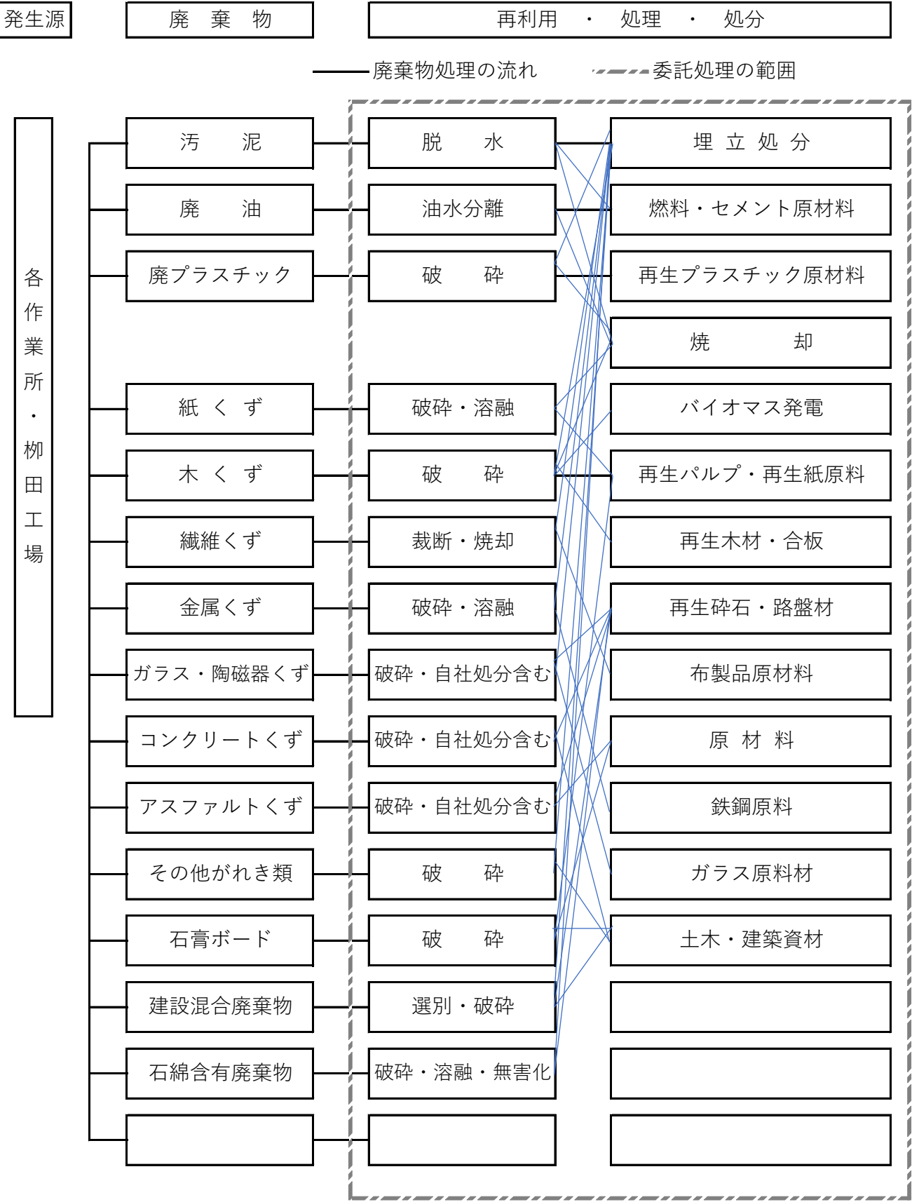
<廃棄物処理フロー図>
