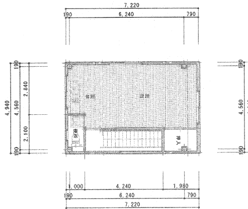
2階平面図 S = 1 : 100
