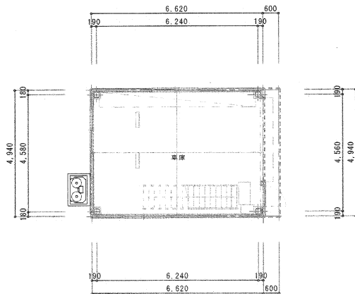
1階平面図 S = 1 : 100
