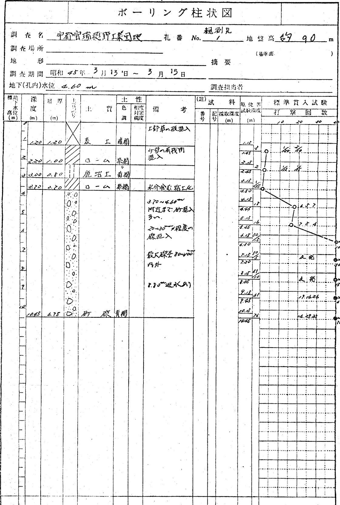
第11図 みずほの園地地盤調査井のくつきく記録 ならびに標準貫入試験結果
