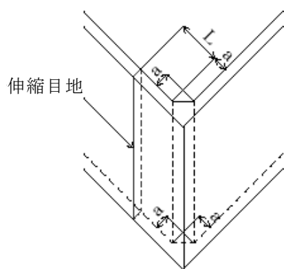
(a)立体図
