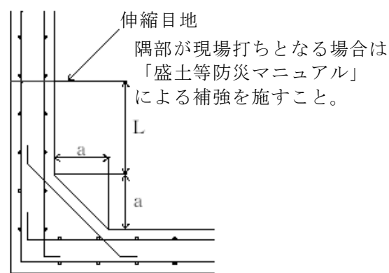
(b)平面図
