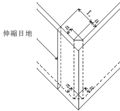
(a)立体図
