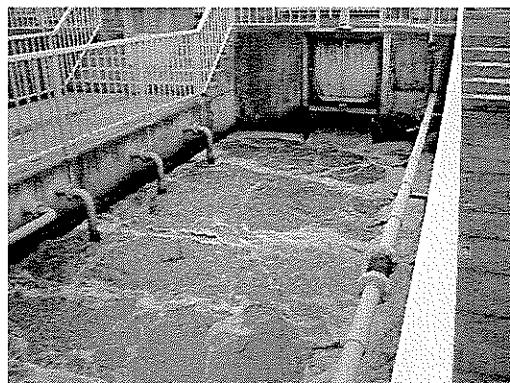
反応タンク（エアレーションタンク）
