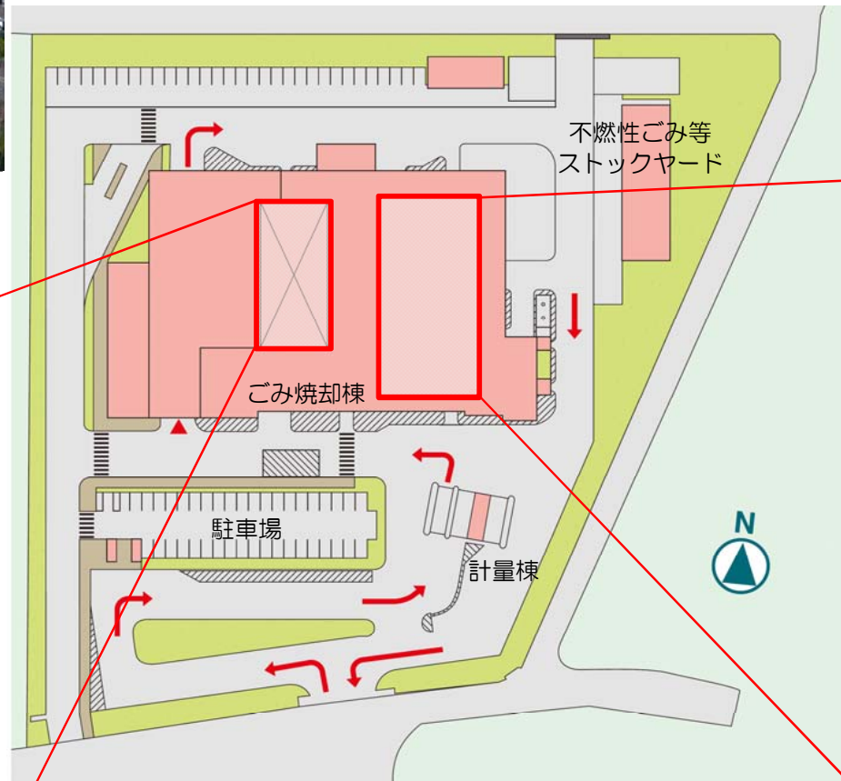
施設全体平面図
