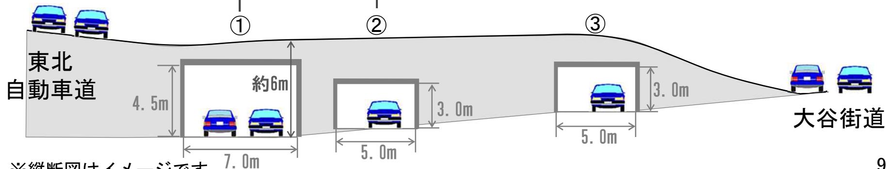
縦断図
