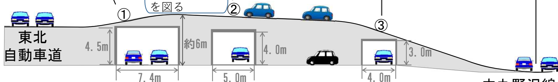
縦断面図
