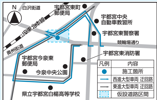
▼工事箇所および大型トラック迂回案内図
