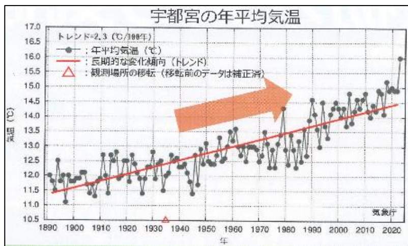
図4.5 100年間で2.3℃上昇（出典：宇都宮気象台・東京管区気象台（令和7年3月））
