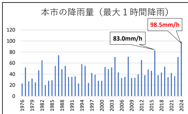
図4.6 本市の最大1時間降雨量の推移
