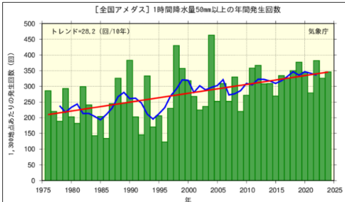
図4.1 1時間降水量 50\text{mm} 以上の年間発生回数の全国的な推移 出典元：気象庁HP
