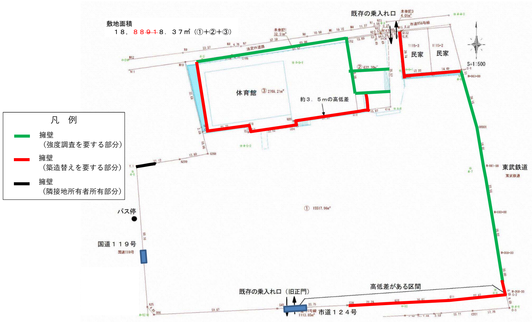
図1 擁壁の取扱い
