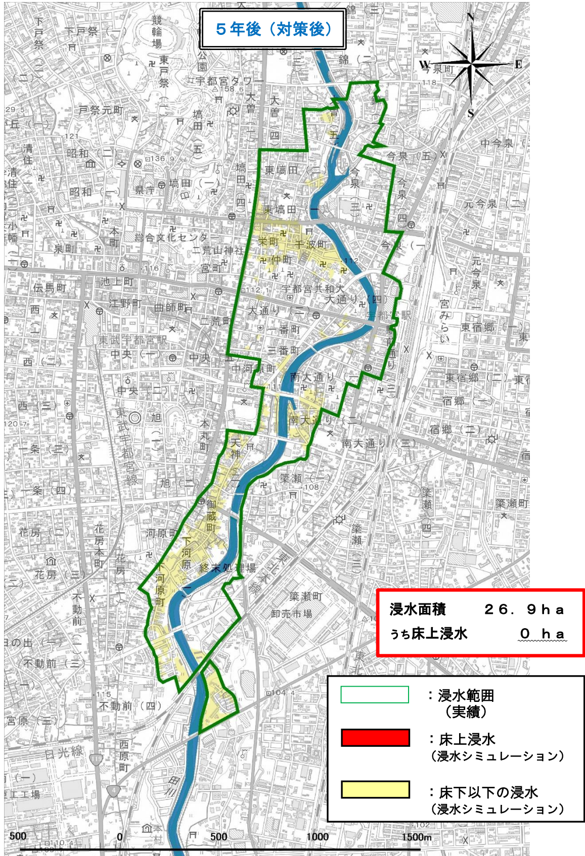
図 5年後(対策後)における田川流域の浸水図(東日本台風の降雨)
