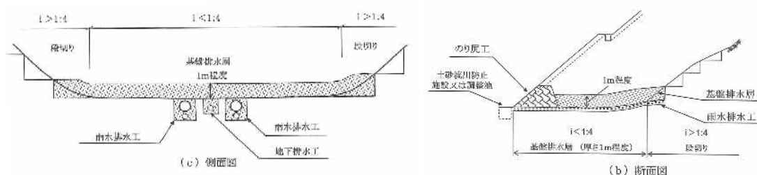
(参考図) 基盤排水層の設置例
