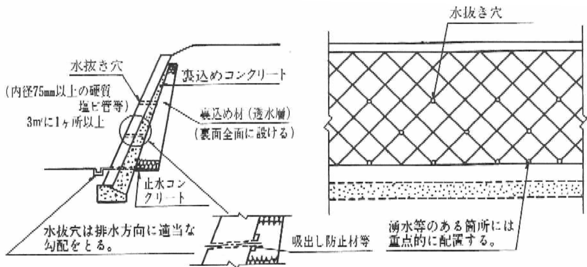
水抜き穴の配置
