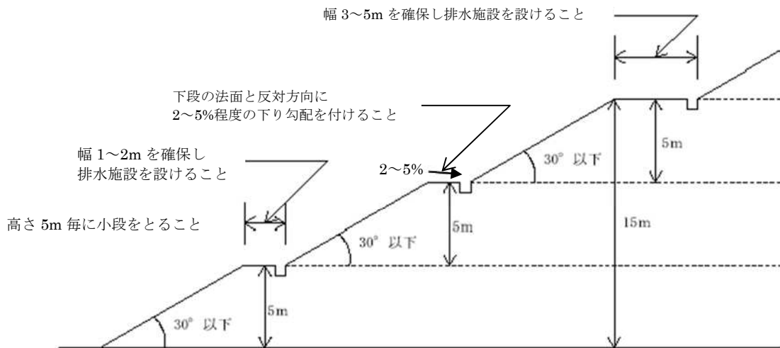
図 1-3 長大法面の保護
