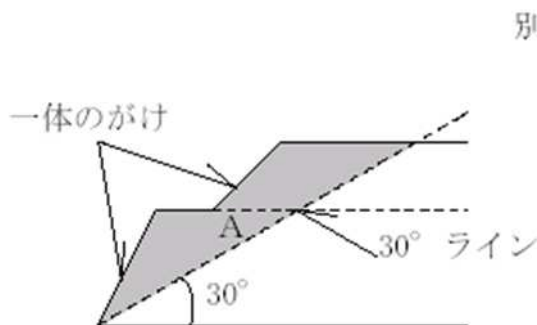
図1-3 一体のがけ
