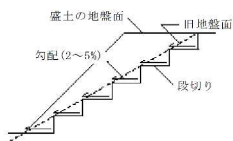
図 1-2 段切り
