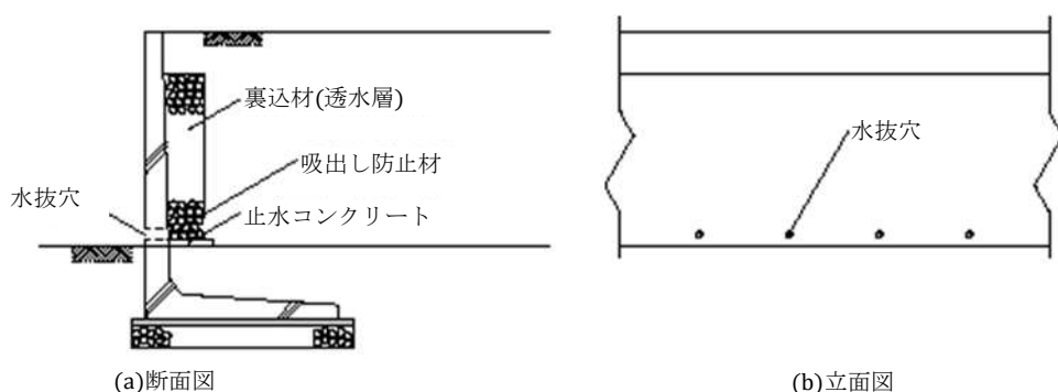
図 5 - 2 水抜き穴の配置図
