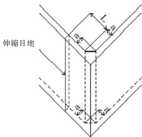
(a)立体図
