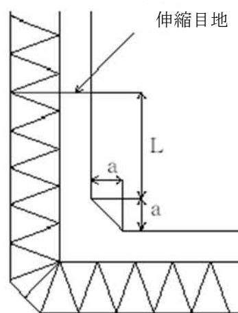
(b)平面図
