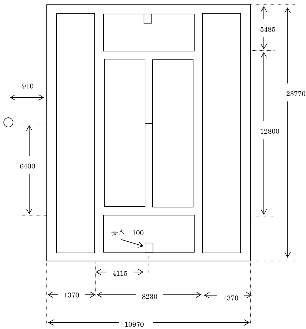
テニスコートライン敷設図
