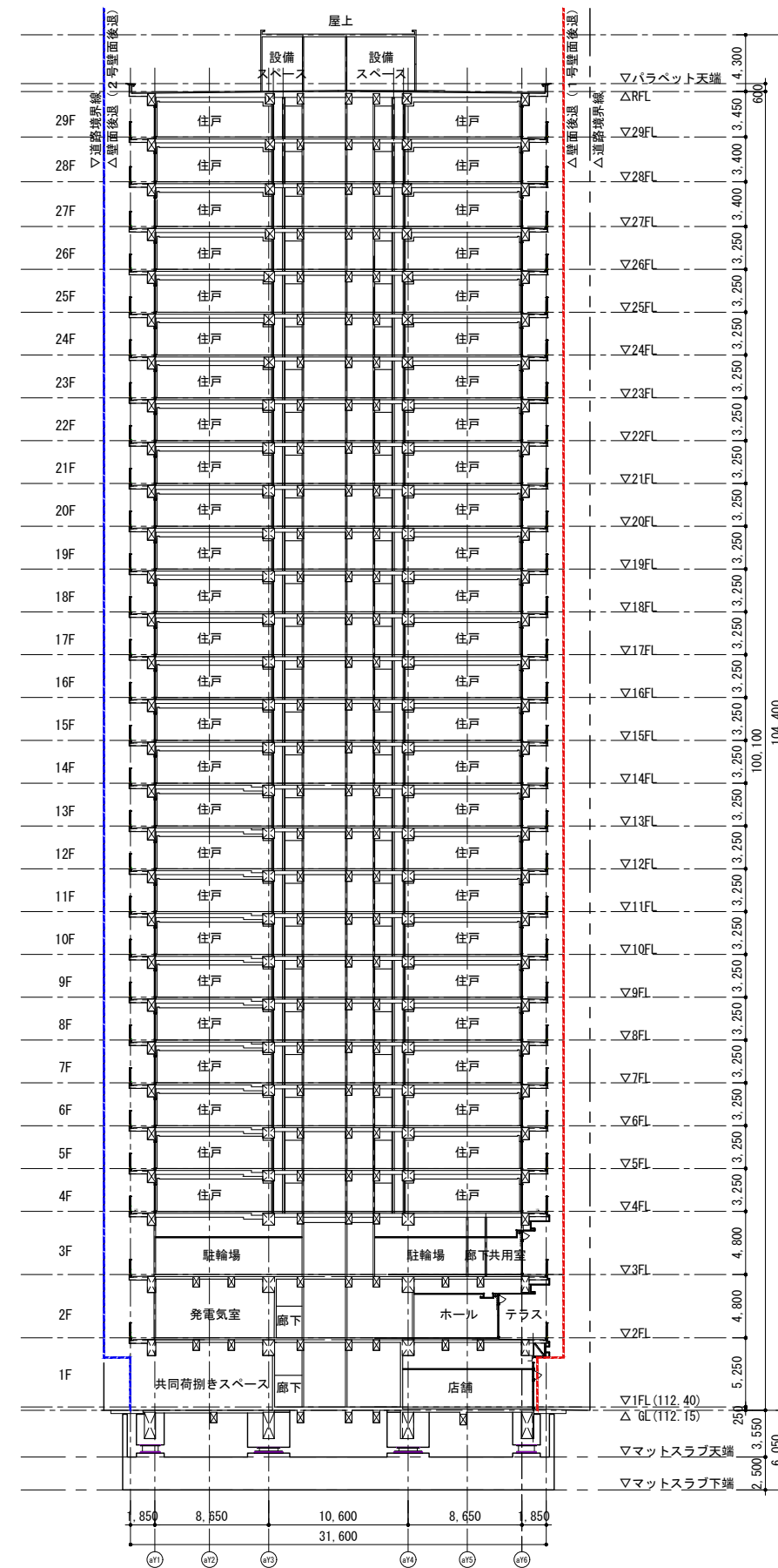
【高層棟南北断面図】
