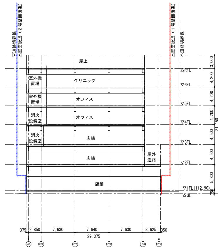
【低層棟南北断面図】
