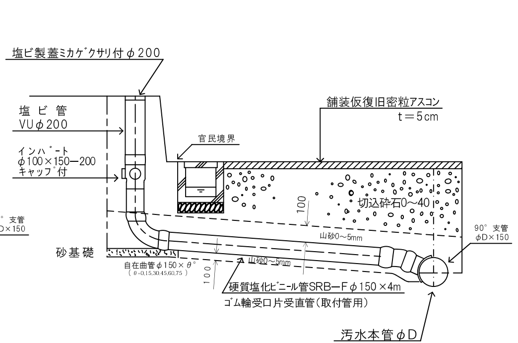
縦型設置の基礎
