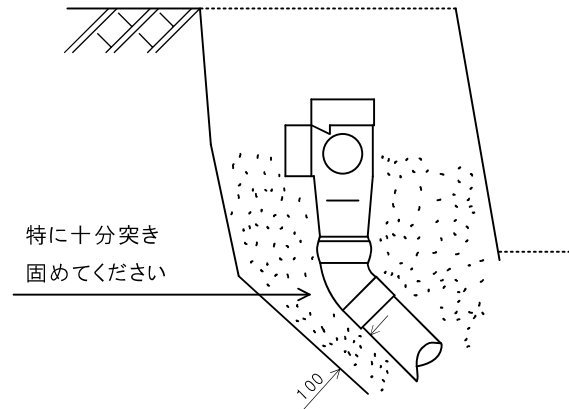
縦型設置の基礎
