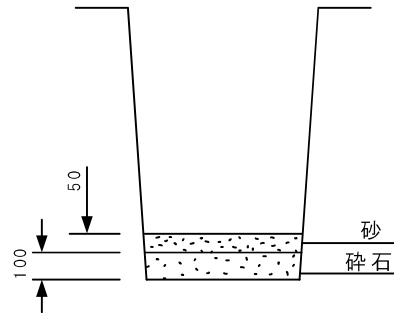
軟弱地盤の基礎
