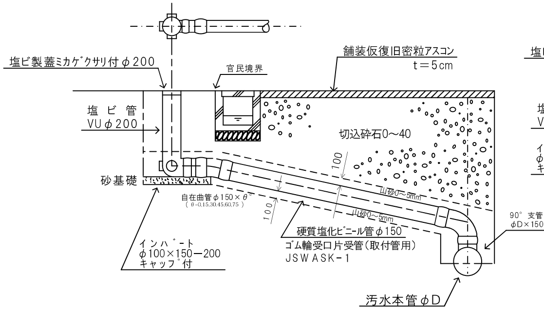
横型・90° 三方合流
