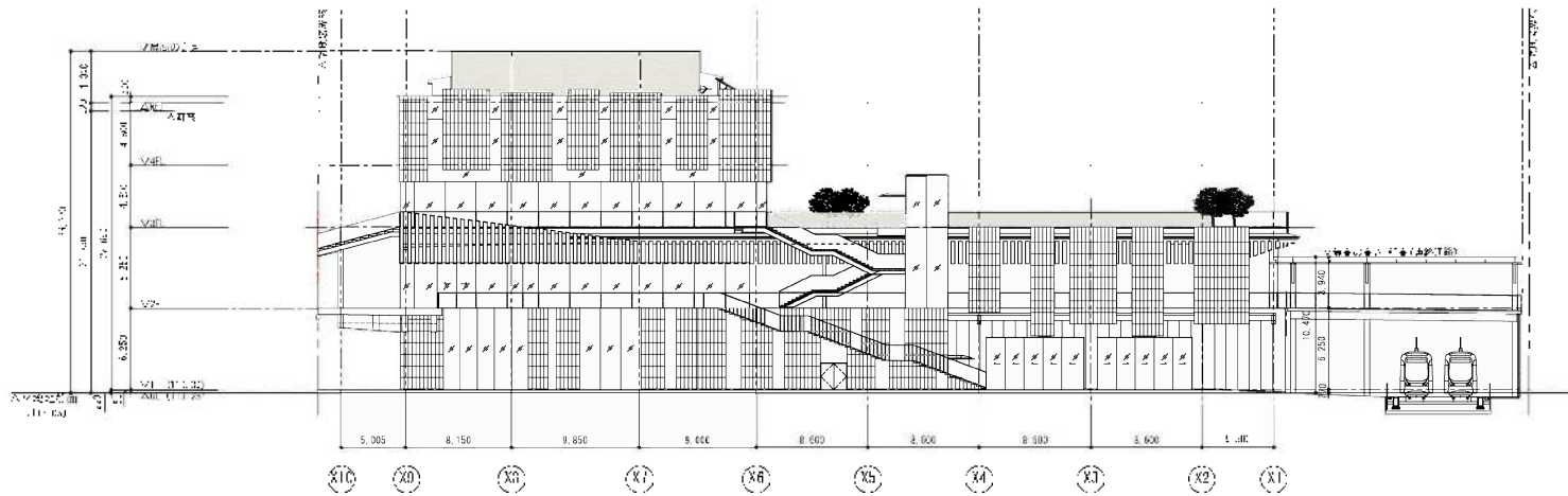
西侧立面图
